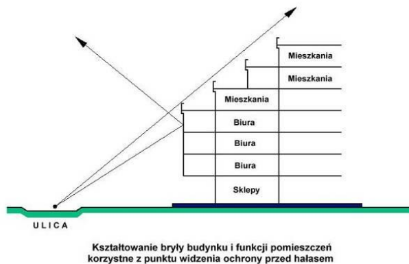
Rysunek 21. Przykład rozmieszczenia pomieszczeń w budynku.
